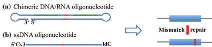
圖三 寡核苷酸標靶突變
