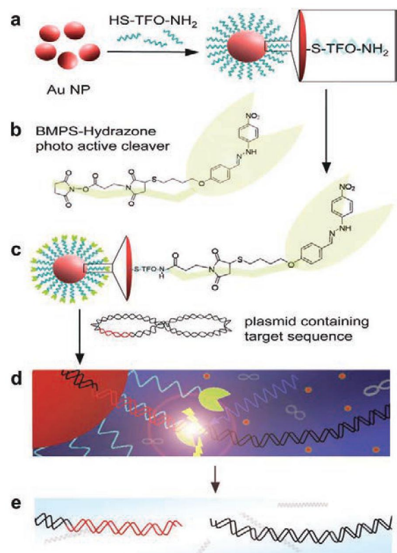
(a) 特定TFOs分子聚集在金奈米粒子。 (b) BMPS-hydrazone 結合上TFO。 (c) TFOs分子識別目標DNA質體且形成穩定的鍵結。 (d) 當暴露在紫外線光，hydrazone造成DNA雙鏈斷裂。 資料來源：Tsai, 2010。
